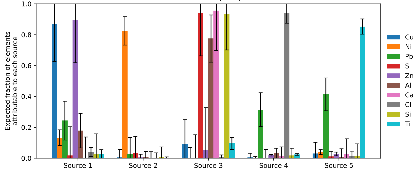
GeomNMF (K=5)
