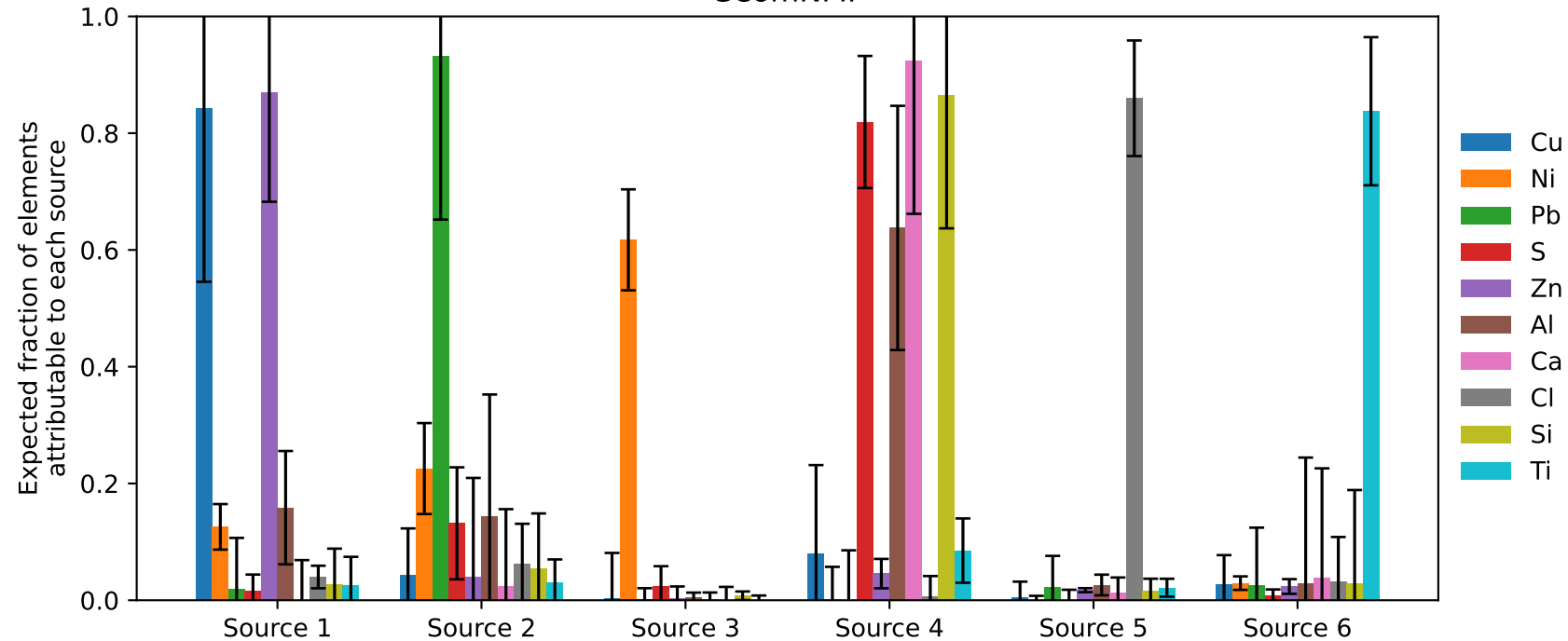
GeomNMF
