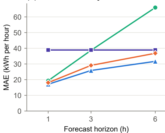
(d) BDG2 electricity
