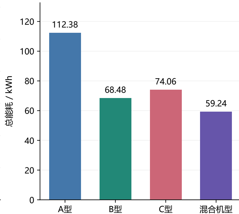
统一机型与混合机型方案比较 (均完成全部货物运输)
