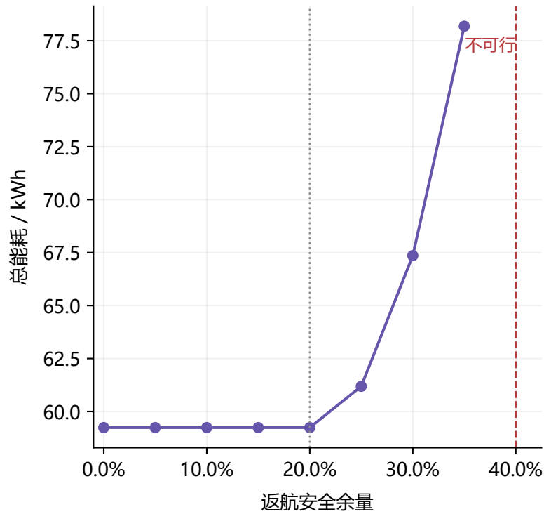
混合机型方案随安全余量的变化（离散情景比较）
