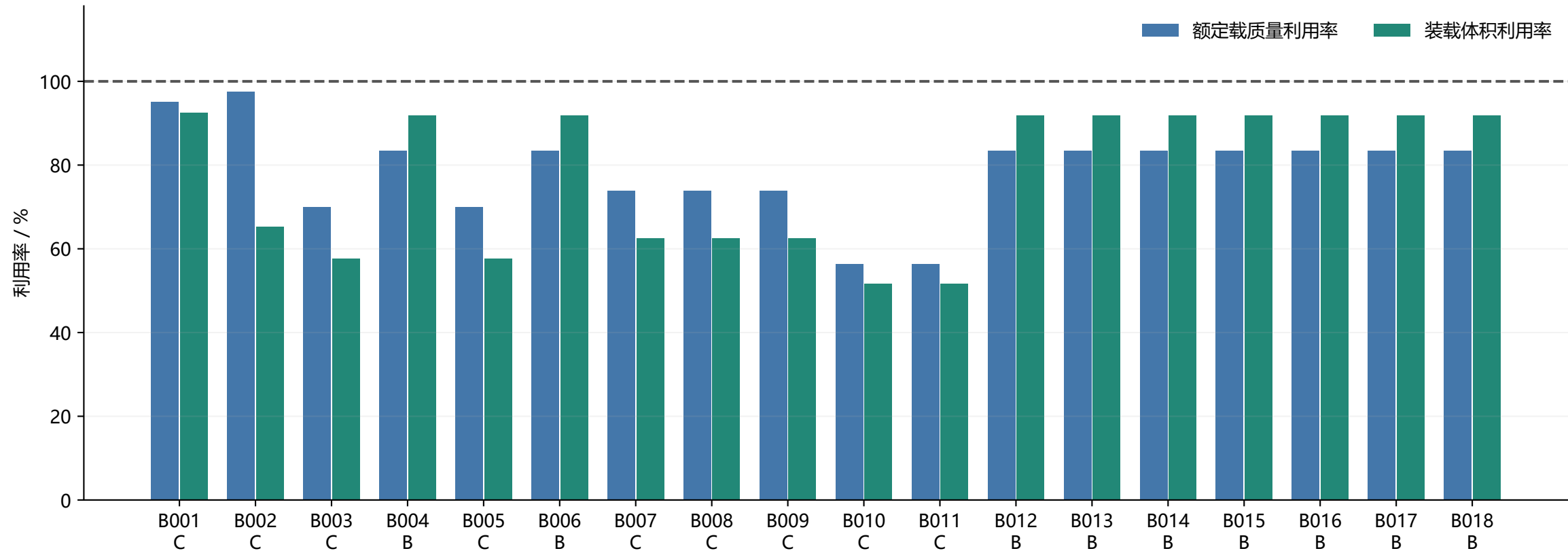
逐架次质量与体积约束利用率
