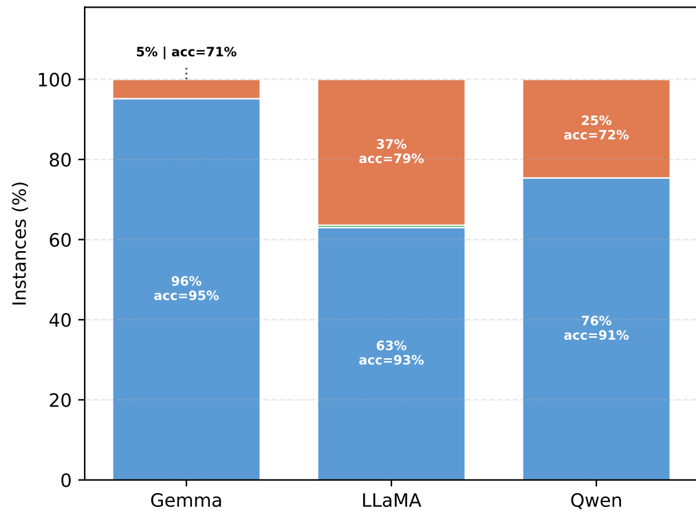
PrOntoQA
