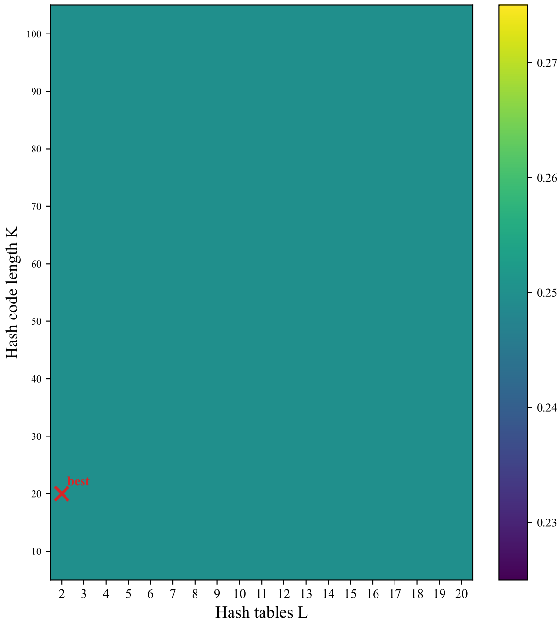
cifar10: Precision
