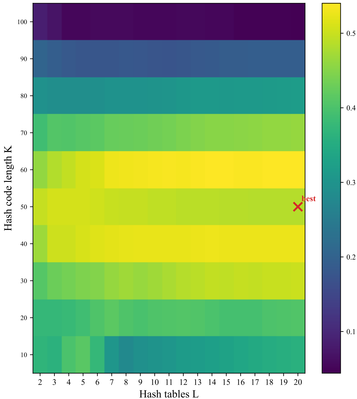
isolet: F1
