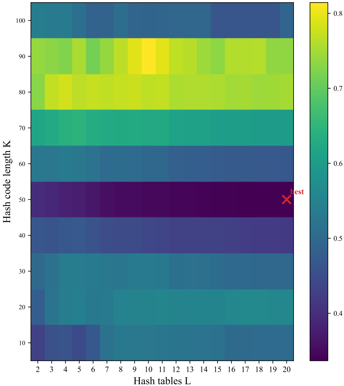
isolet: Precision
