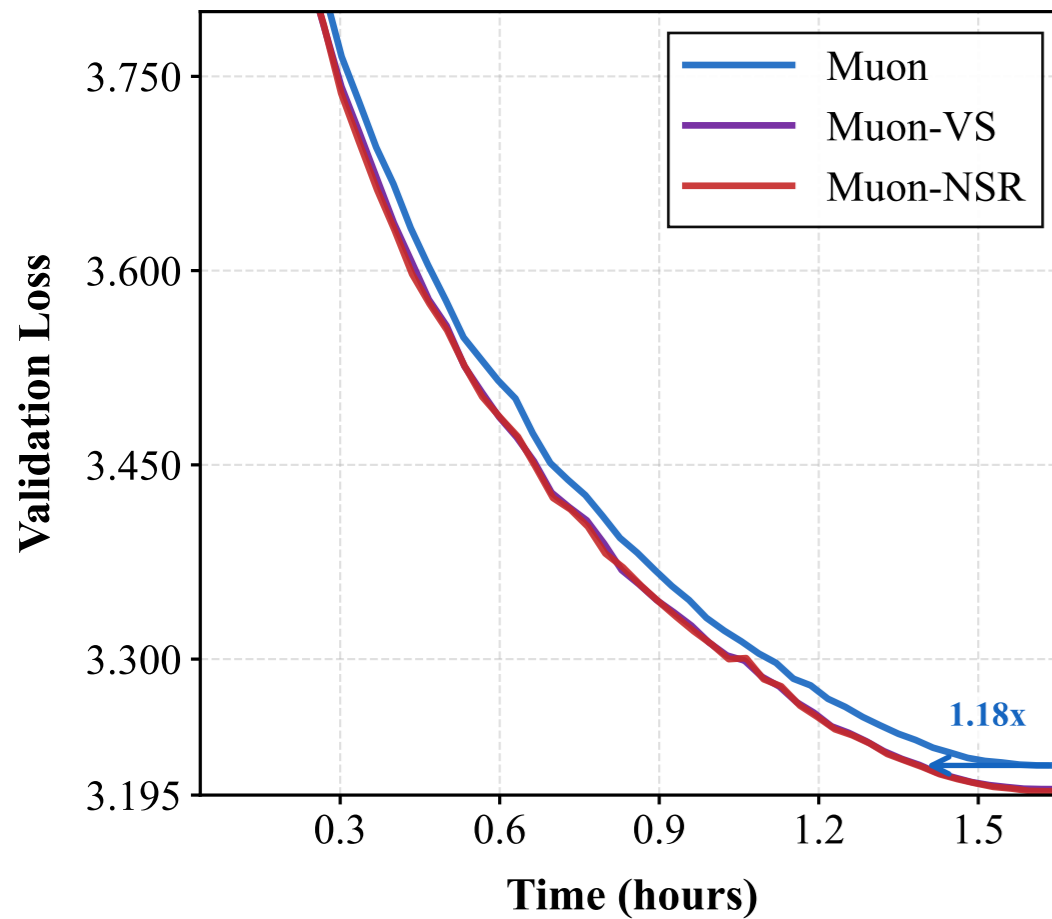
Llama - 130M
