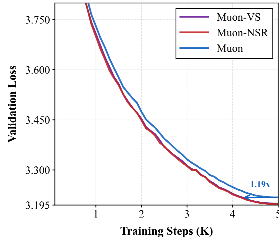
Llama - 130M
