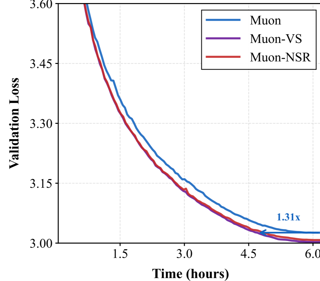
Llama - 300M
