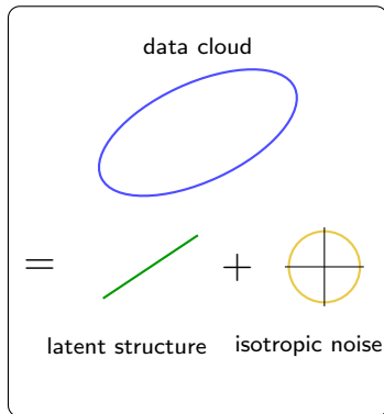
PPCA
