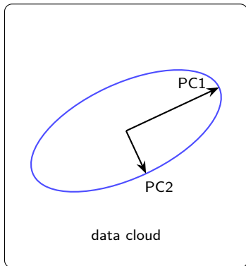
PCA
