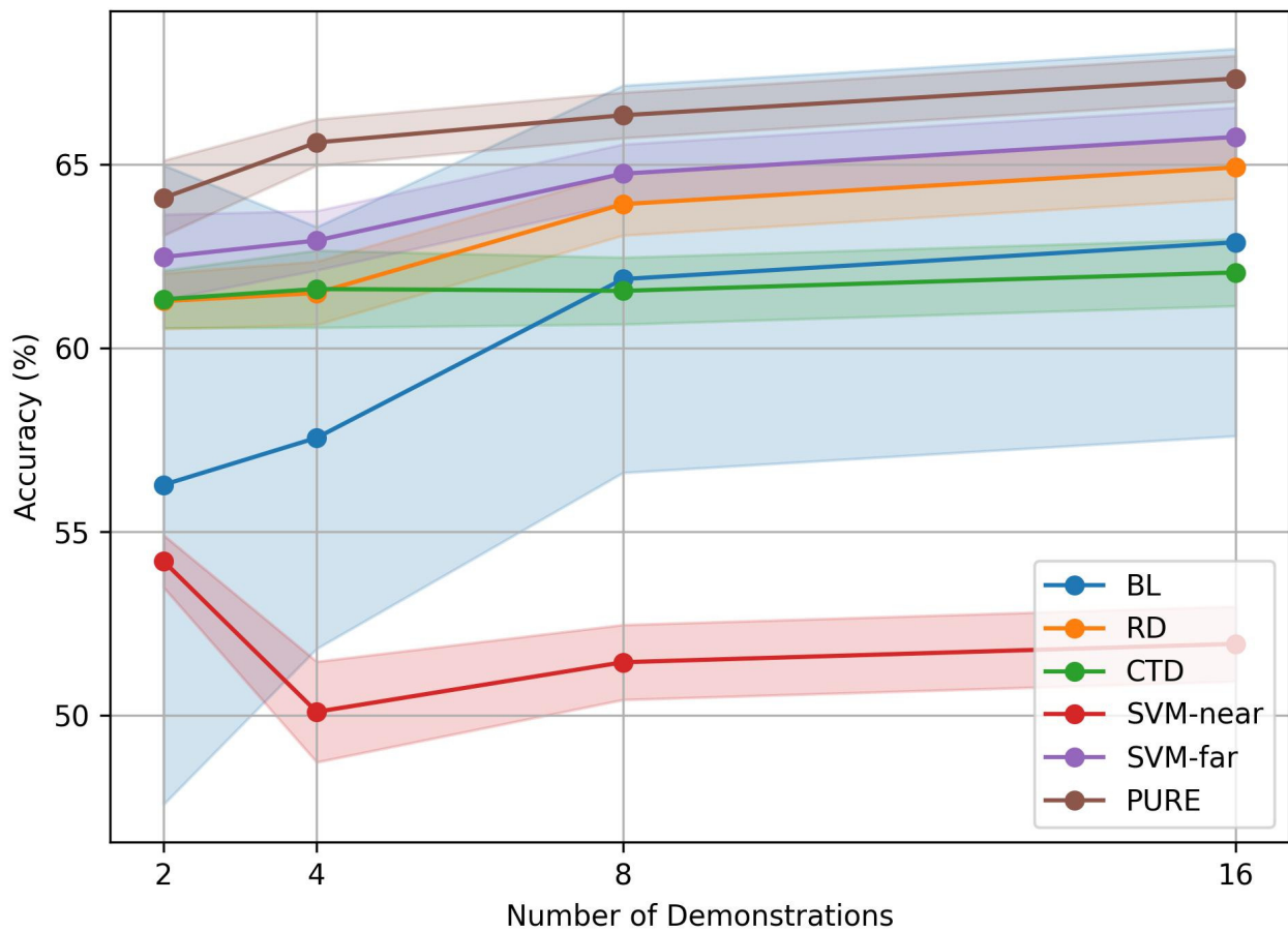
BNCI2014001
