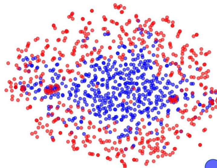
T-SNE
