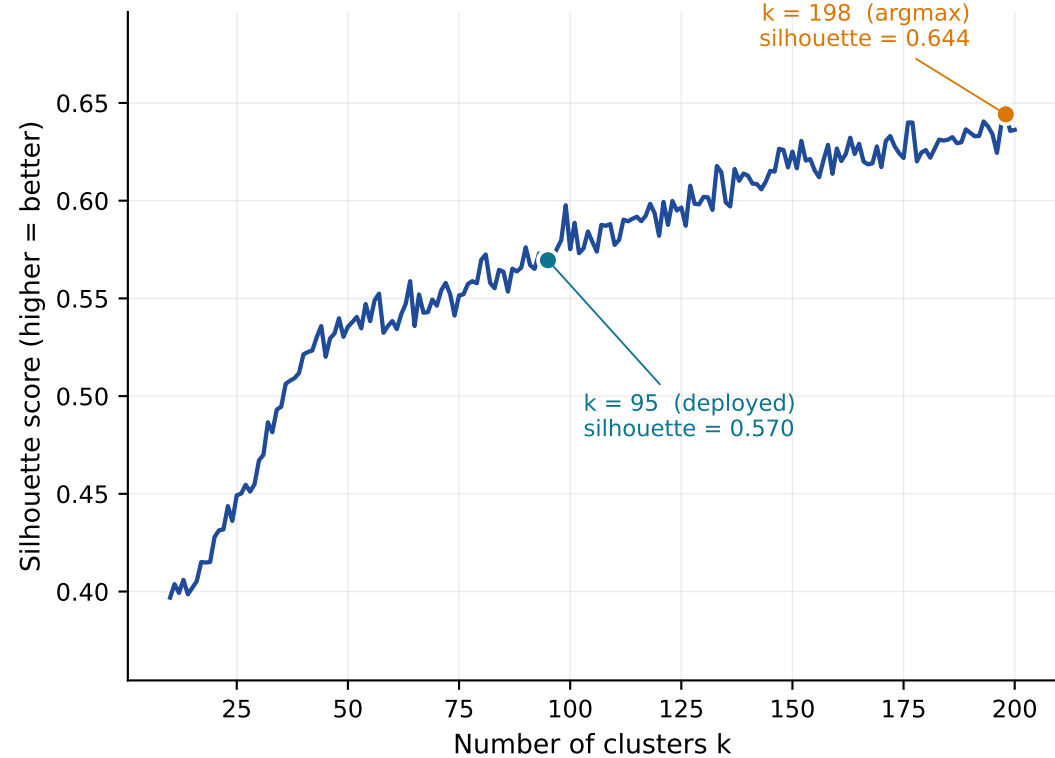
A. Silhouette
