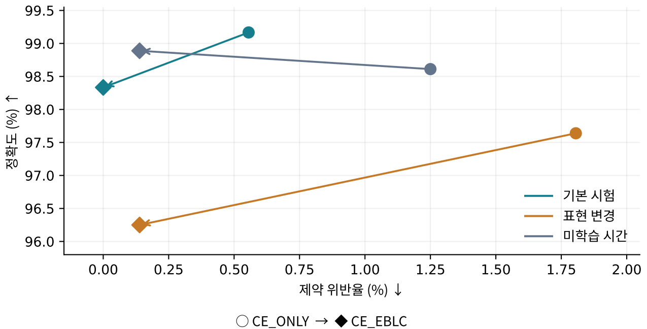
그림 S1. 동일 평가 조건의 CE_ONLY에서 CE_EBLC로 향하는 화살표이다. 가로축 위반율은 낮을수록, 세로축 정확도는 높을수록 좋다. 점은 세 시드 평균이며 연결은 학습 궤적이 아니라 두 학습 조건의 비교이다. 작은 차이를 보이기 위해 두 축을 확대했다.
