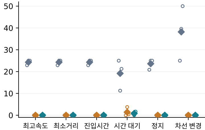
위반율 (%) ↓
