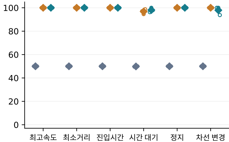
정확도 (%) ↑
