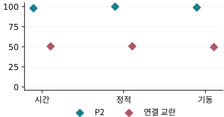
정상 연결 / 학습 연결 교란 정확도 (%)
