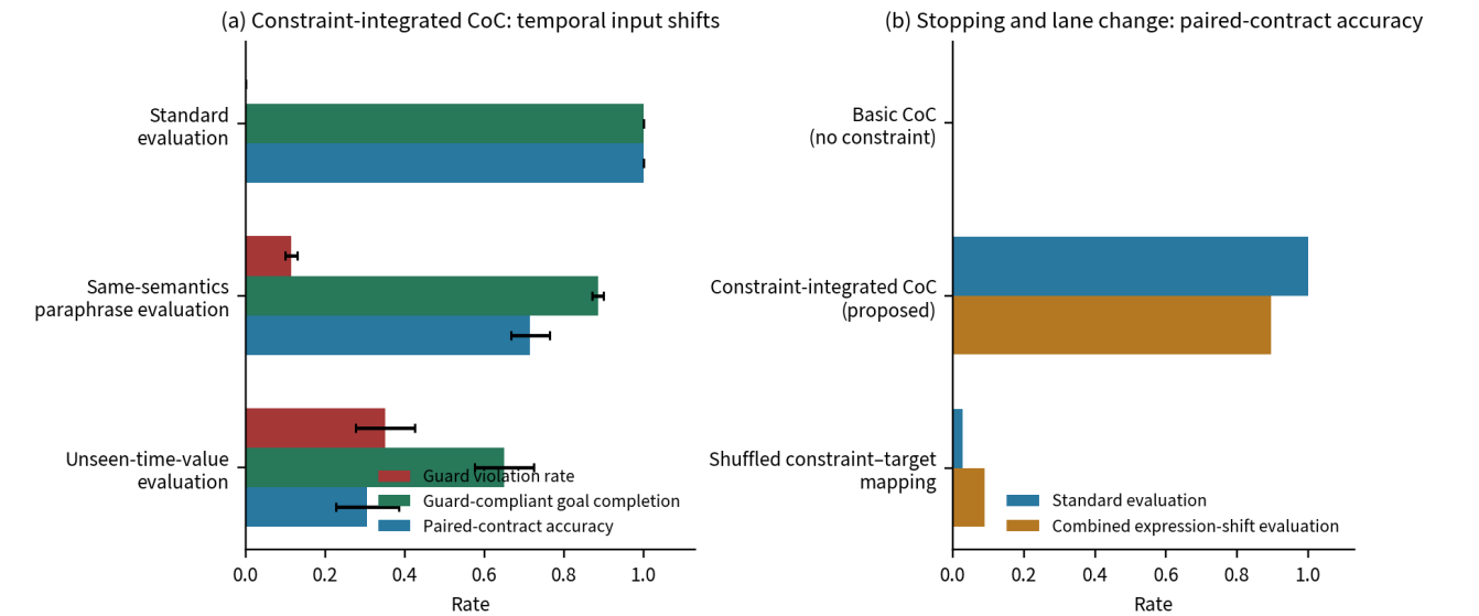
그림 5. 입력 변화에 따른 성능. (a)는 제약 통합 CoC의 시간 과제를 비교한다. 빨간색 가드 위반률은 낮을수록, 초록색 가드 준수 목표 완료율과 파란색 계약 쌍 정확도는 높을수록 좋다. 표준 평가에서는 위반률 0.000, 나머지 두 지표 1.000이지만 동일 의미 문장 변형 평가에서 낮아지고, 미관측 시간값 평가에서 가장 크게 낮아진다. (b)는 정지·차선 변경 과제의 계약 쌍 정확도다. 파란색은 표준 평가, 주황색은 경계·부정·순서·단위 변화가 함께 든 복합 표현 변화 평가다. 기본 CoC와 대응 교란 통제군은 낮고 제약 통합 CoC만 두 평가에서 높은 값을 유지한다. (a)의 오차 막대는 모집단 표준편차이며 (b)의 표 값은 표본 표준편차를 사용한다. Fig. 5. Performance under input shifts. Panel (a) shows temporal degradation from standard to paraphrased and unseen-time evaluations; panel (b) compares paired-contract accuracy under standard and combined expression shifts.
