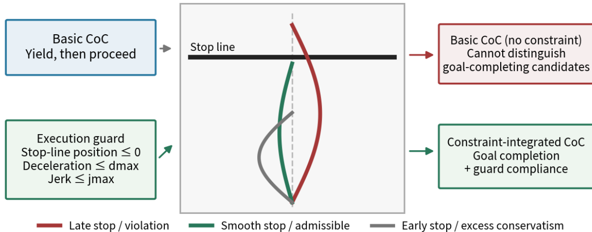
그림 1. 기본 CoC와 제약 통합 CoC의 선택 기준 차이. 세 후보는 모두 '보행자에게 양보한 뒤 진행'이라는 목표와 관련되지만, 빨간 궤적은 정지선, 동역학 제약을 위반하고 회색 궤적은 허용되지만 지나치게 보수적이다. 기본 CoC만으로는 두 실행 품질을 구별하기 어렵고, 제약 통합 CoC는 목표를 완료하면서 제약을 지키는 녹색 후보를 선택할 기준을 제공한다. Fig. 1. Difference between basic CoC and constraint-integrated CoC: the latter distinguishes violating, overly conservative, and admissible goal-completing candidates.
