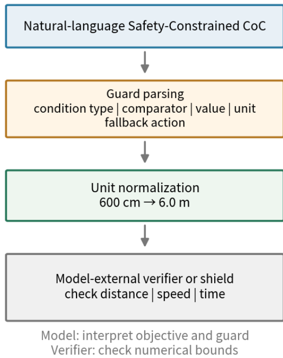
그림 7. 자연어 실행 가드를 실제 검사에 연결하는 네 단계. 위에서 아래로 (1) 자연어 제약 통합 CoC를 읽고, (2) 조건 종류, 비교 방향, 값, 단위, 대체 행동으로 나누며, (3) 600 cm를 6.0 m처럼 기존 단위로 통일하고, (4) 모델 외부 검증기 또는 차단장치가 선택한 제계의 거리, 속도, 시간을 수치 경계와 비교한다. 모델은 목표와 가드를 해석하고 결정적 검증기는 정확한 수치 판정을 담당한다.
