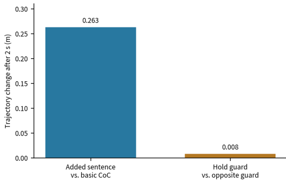
그림 4. Alpamayo-R1 사전 진단. 첫 막대 0.263 m는 문장을 추가했을 때 기본 CoC와 달라진 정도이므로 '추가 문장에 대한 반응'을 나타낸다. 두 번째 막대 0.008 m는 대기 가드와 반대 가드의 차이이므로 '반대 의미의 구별'을 나타낸다. 두 번째 값이 매우 작아 이 한 장면만으로 의미에 맞는 가드 준수를 확인할 수 없다.
