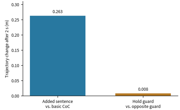
그림 4. Alpamayo-R1 사전 진단. 첫 막대 0.263 m는 문장을 추가했을 때 기본 CoC와 달라진 정도이므로 '추가 문장에 대한 반응'을 나타낸다. 두 번째 막대 0.008 m는 대기 가드와 반대 가드의 차이이므로 '반대 의미의 구별'을 나타낸다. 두 번째 값이 매우 작아 이 한 장면만으로 의미에 맞는 가드 준수를 확인할 수 없다.
