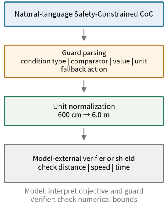
그림 7. 자연어 실행 가드를 실제 검사에 연결하는 네 단계. 위에서 아래로 (1) 자연어 제약 통합 CoC를 읽고, (2) 조건 종류·비교 방향·값·단위·대체 행동으로 나누며, (3) 600 cm를 6.0 m처럼 기준 단위로 통일하고, (4) 모델 외부 검증기 또는 차단장치가 선택한 궤적의 거리·속도·시간을 수치 경계와 비교한다. 모델은 목표와 가드를 해석하고 결정적 검증기는 정확한 수치 판정을 담당한다.
