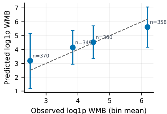
TCGA→CPTAC: calibration bins
