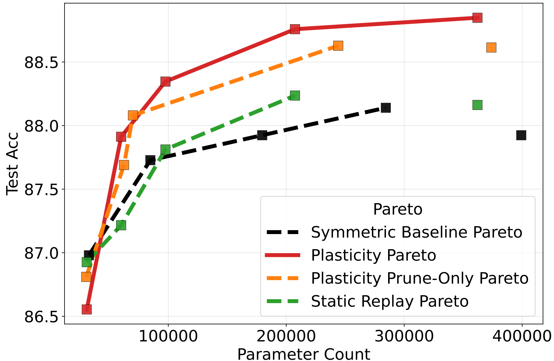
Test Acc vs Parameter Count
