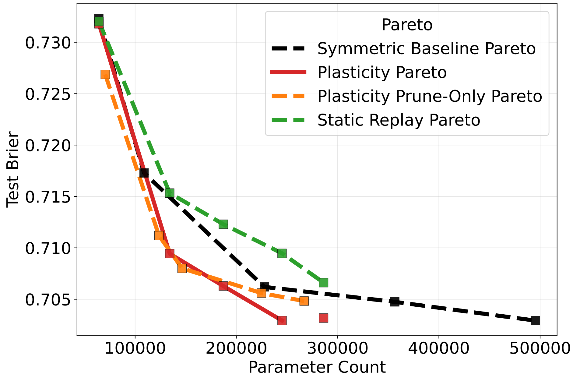
Test Brier vs Parameter Count
