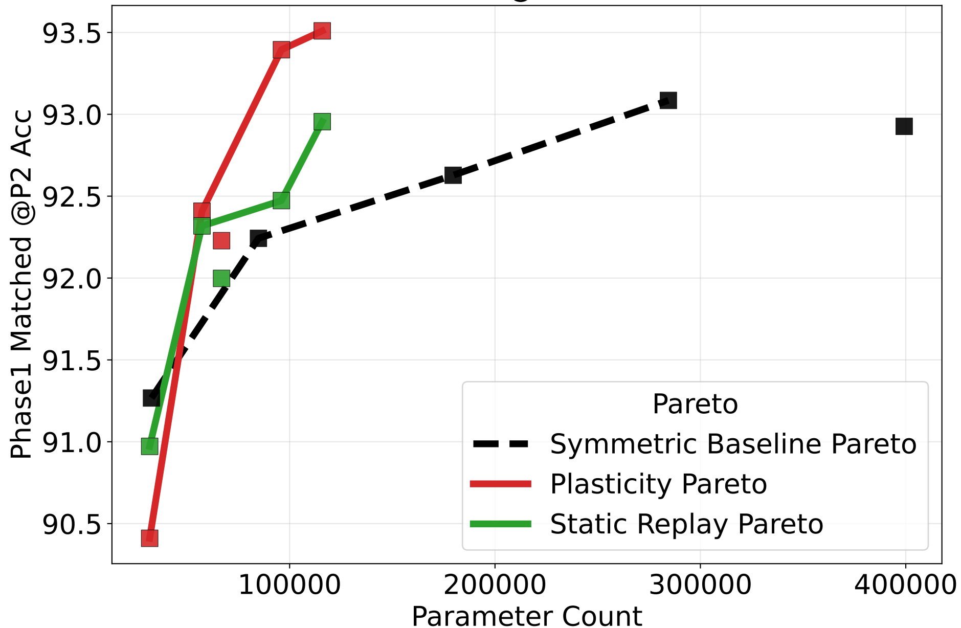
Phase-1 Matched Acc @P2 vs Parameter Count
