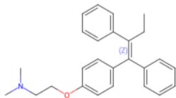
tamoxifen (CID 2733526)
