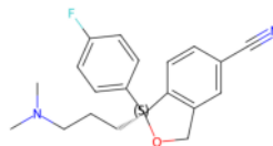
escitalopram (CID 146570)
