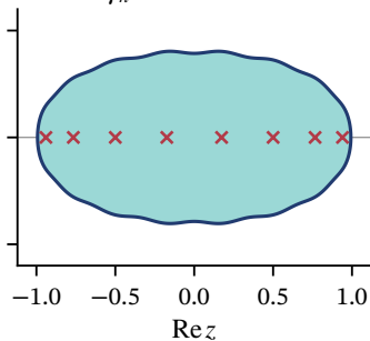
(d) n=8 : connected \hat{\gamma}_n=0.0038 < \varepsilon
