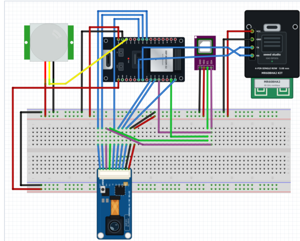
[그림 1] ESP32 4센서 결선도. 좌측 표의 핀 배정과 1:1로 대응한다.
