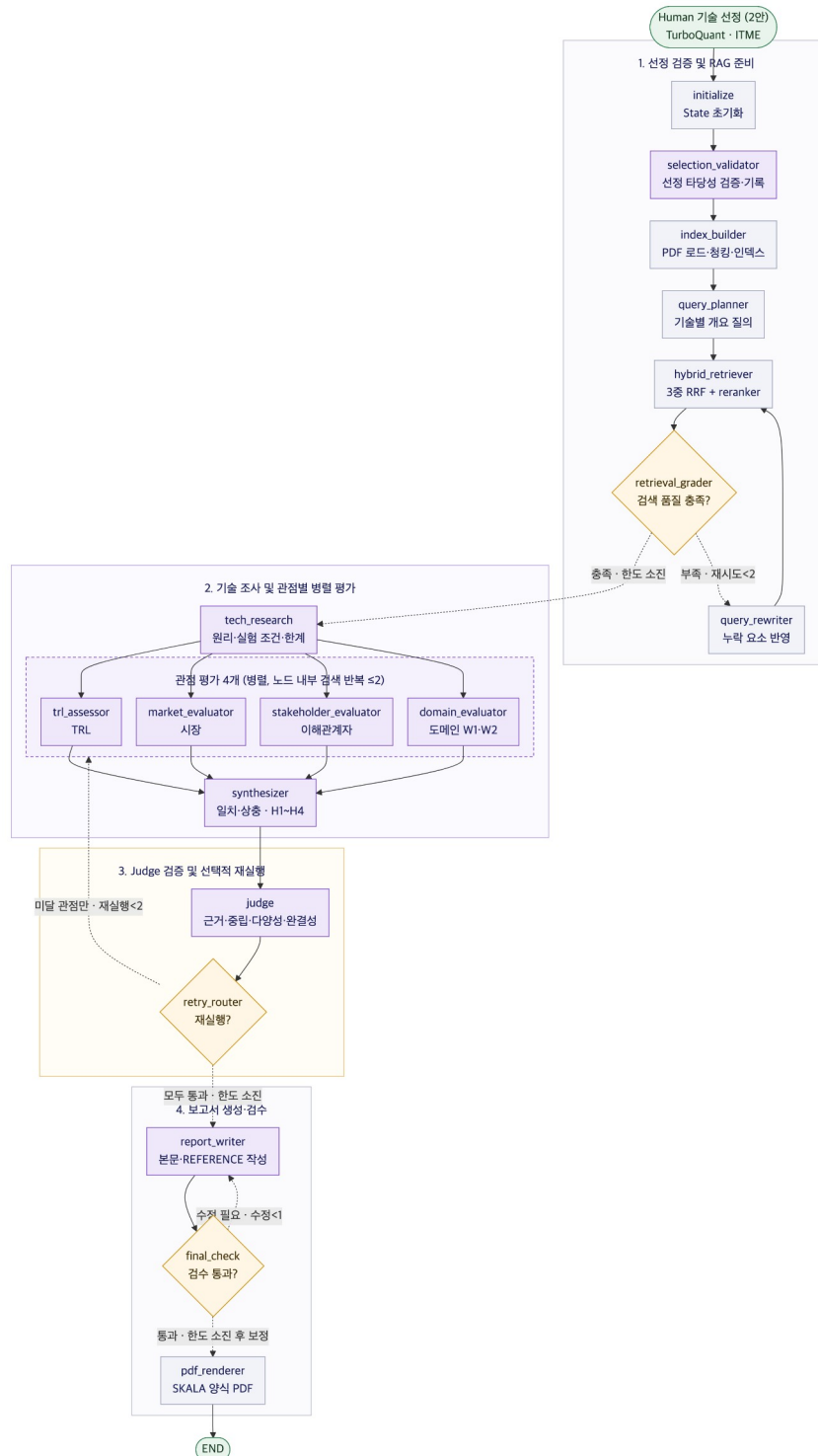
그림 2. 전체 그래프(노드 18개). 실선은 항상 지나는 경로, 점선은 조건에 따라 갈리는 경로이고, 마름모는 다음 경로를 정하는 노드이다
