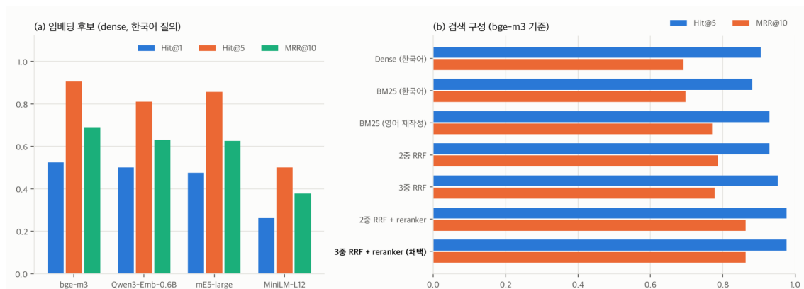
그림 1. 임베딩 후보(a)와 검색 구성(b)의 측정 결과(구현 조건). 출처: 조 자체 측정(42문항 평가셋), eval/run_embedding_eval.py로 측정하고 report/plot_eval_figure.py로 작성
