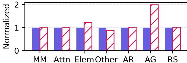
Llama 8B (TP 8 + FSDP 2)
