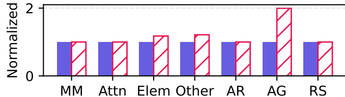
Llama 8B (TP 2 + FSDP 2 + DP 2)
