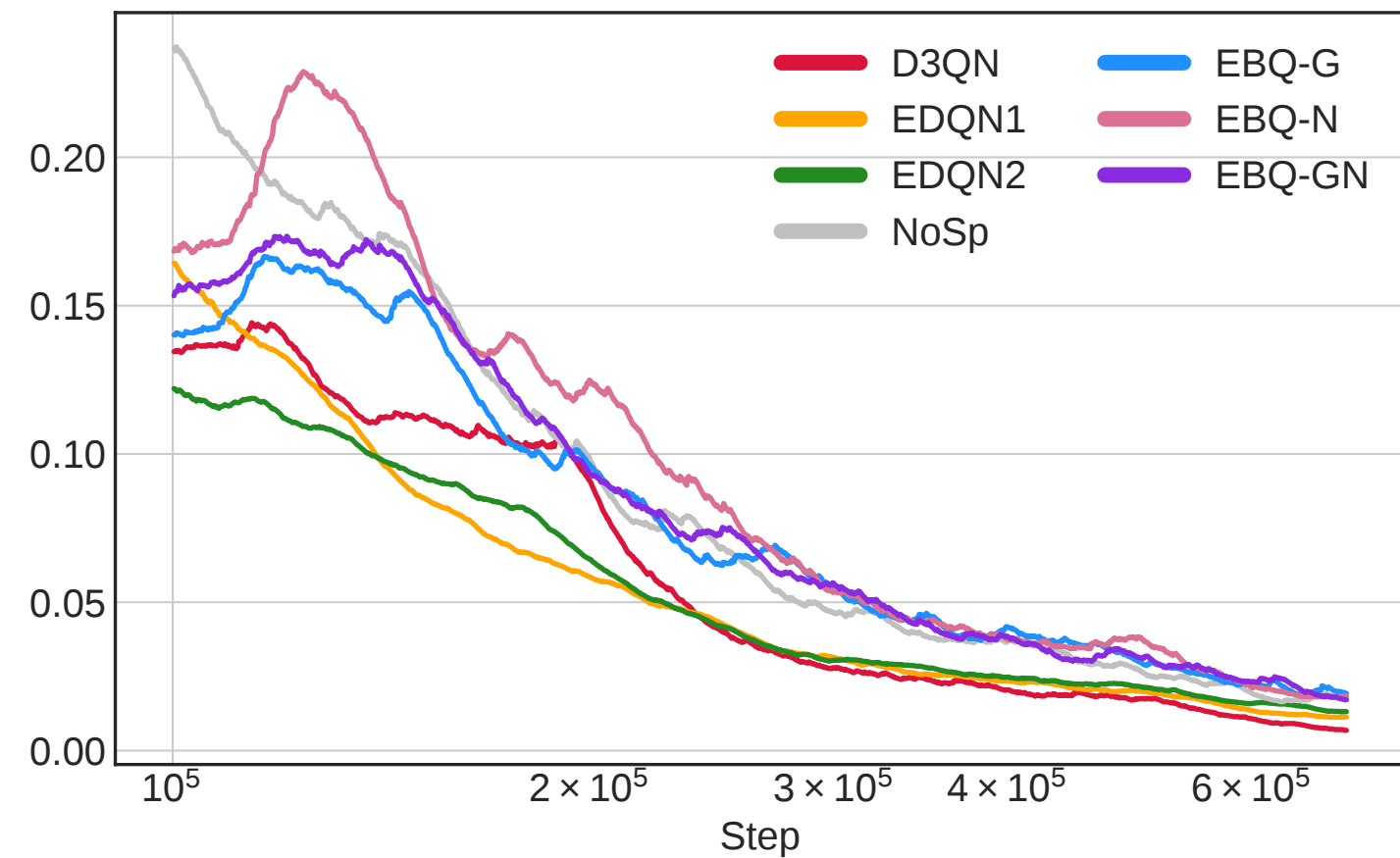
Makespan
