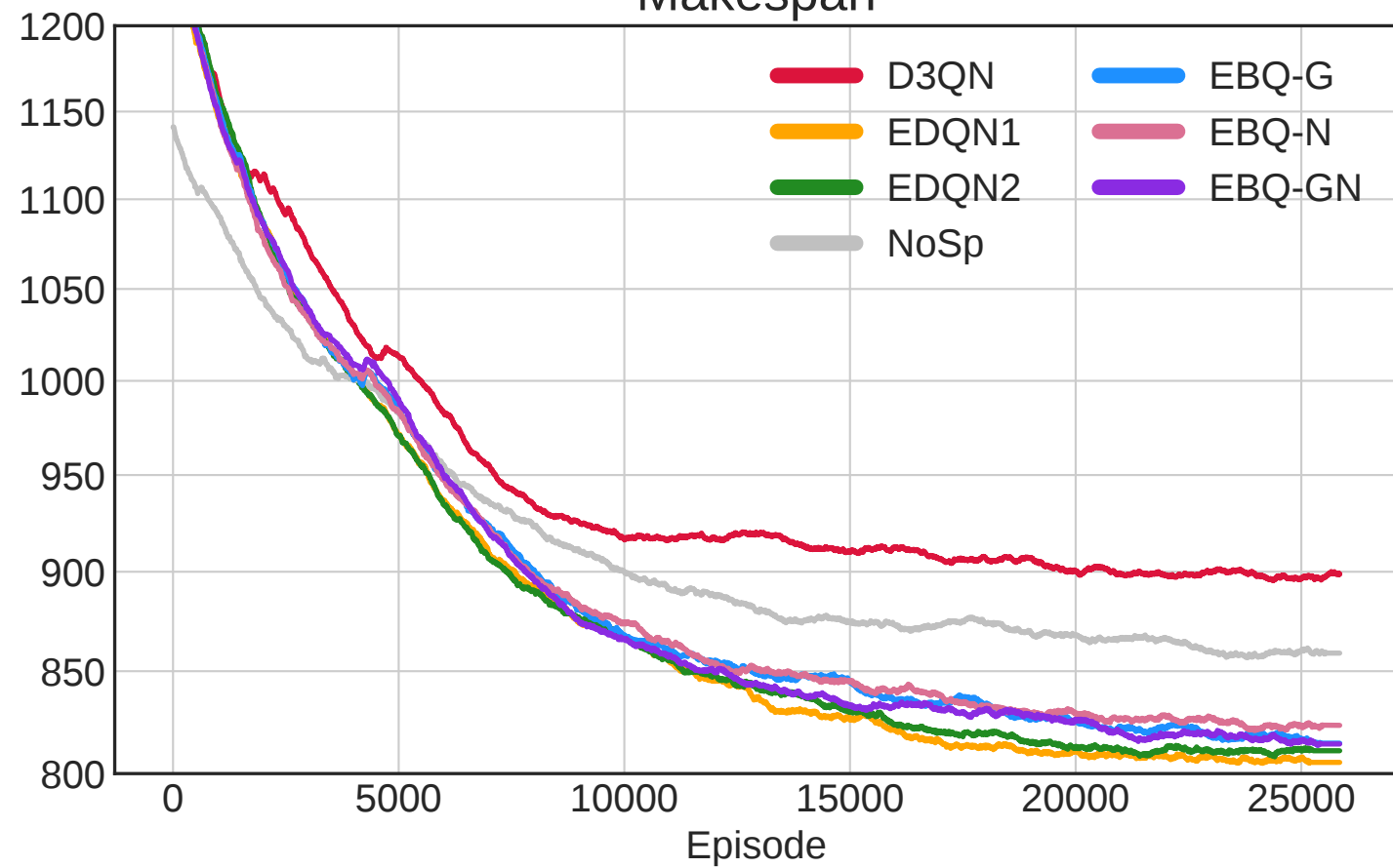
Makespan
