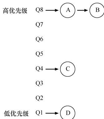
图 8.1 MLFQ 的例子
