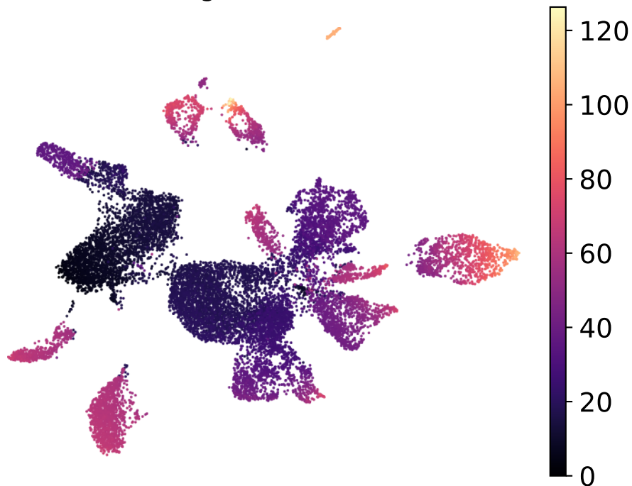
UMAP Slingshot PT (start=11)
