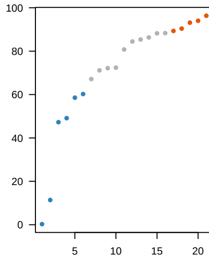
GSE131907
