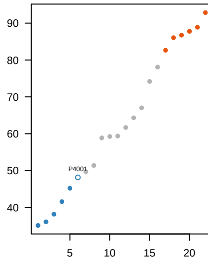
GSE205335
