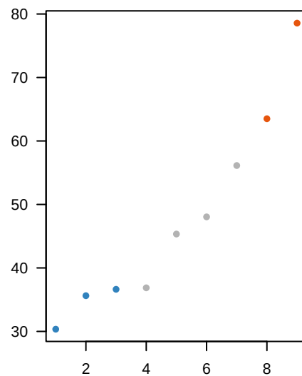
GSE189357
