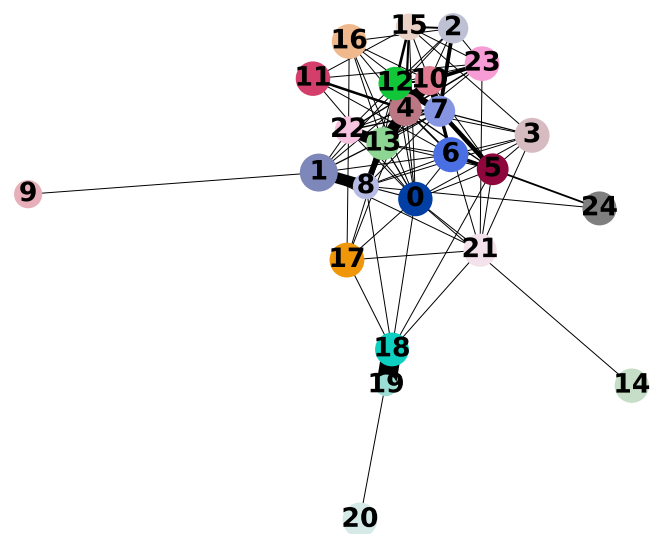
PAGA 1 component(s)
