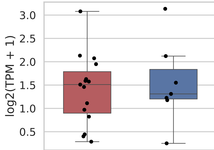
CLDN4
