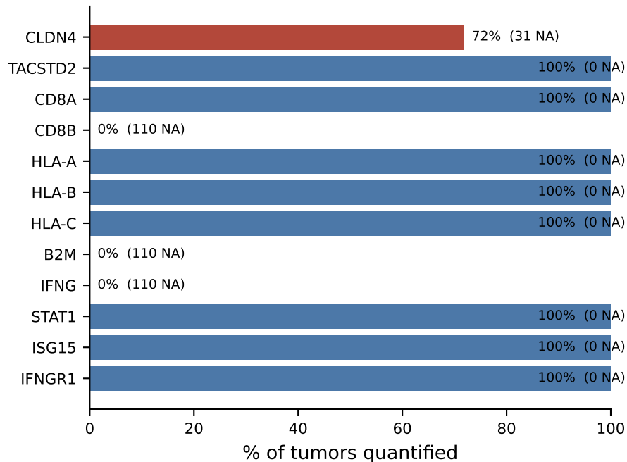
LUAD (n=110)
