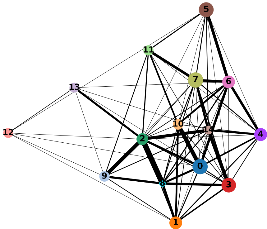
PAGA (Leiden)
