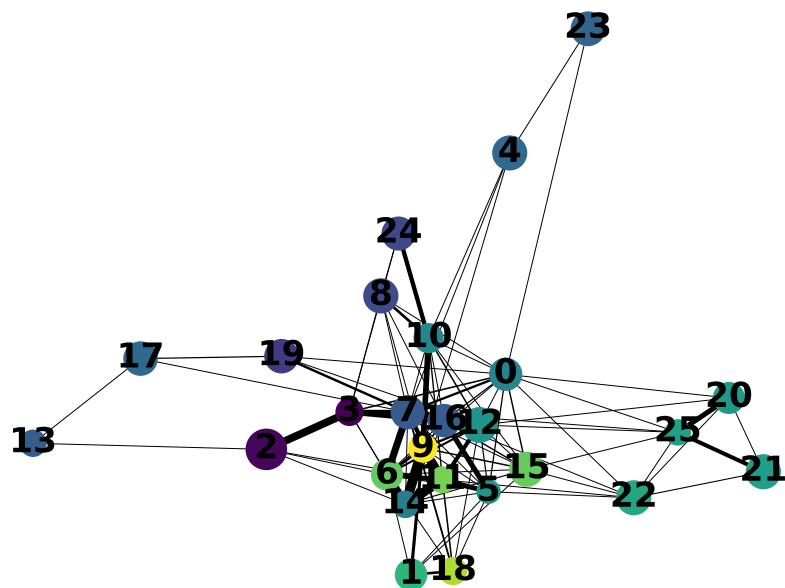
GSE205335 PAGA mean CLDN4
