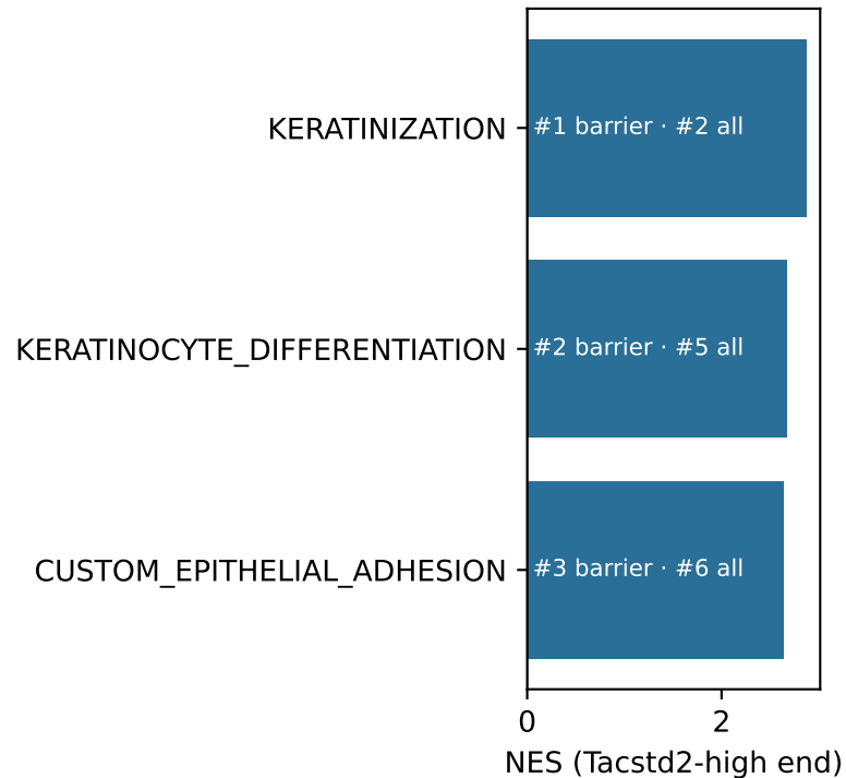
concordant4 malignant
