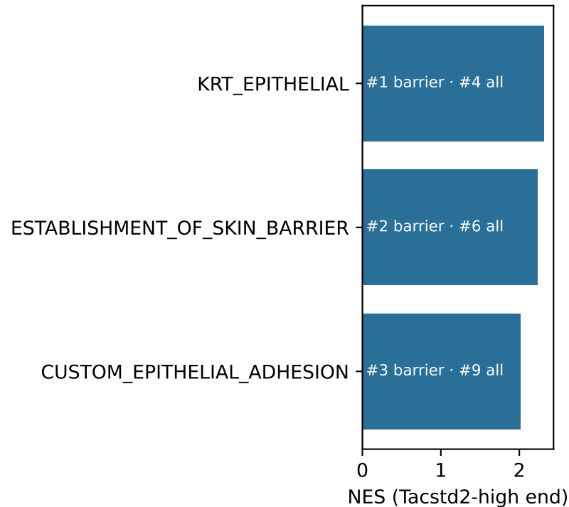
OncoSG LUAD
