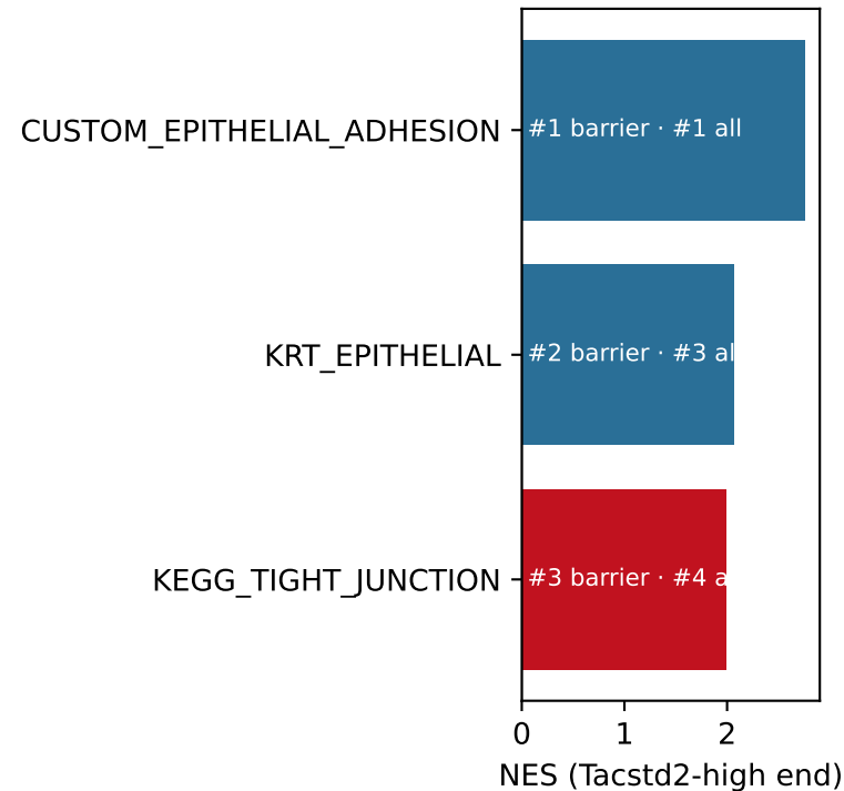
GSE31210 LUAD
