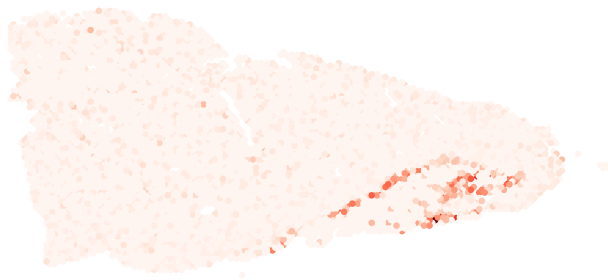
10x_NSCLC_NEC_11mm CLDN4 (log CP10k)
