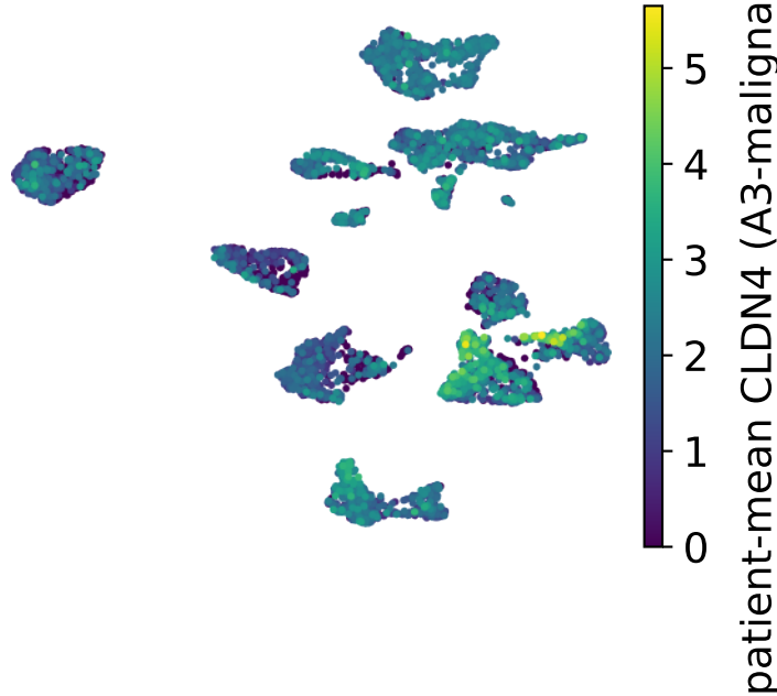
UMAP CLDN4
