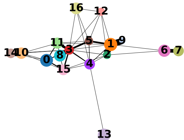
PAGA (Leiden)
