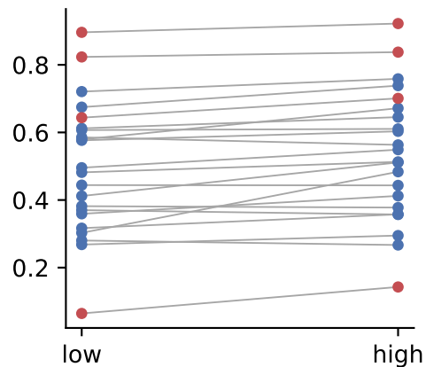
HLA-B_CD8A n=22
