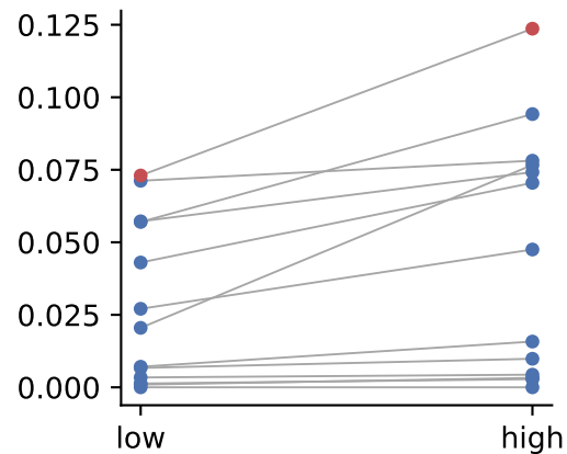
HLA-B_CD8A n=22
