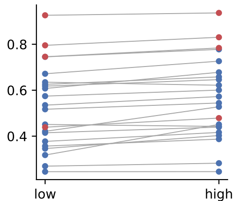
HLA-A_CD8A n=22
