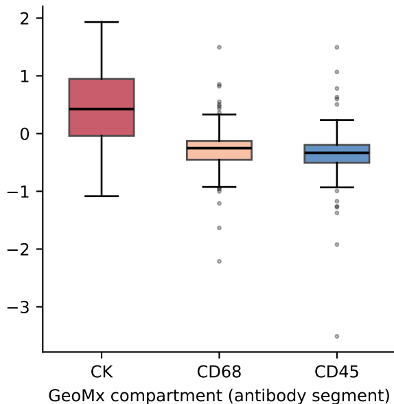
CLDN4/TACSTD2 score
