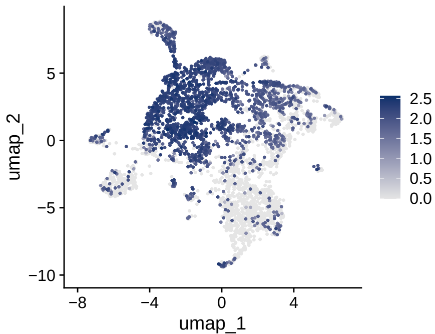
MHC_module
