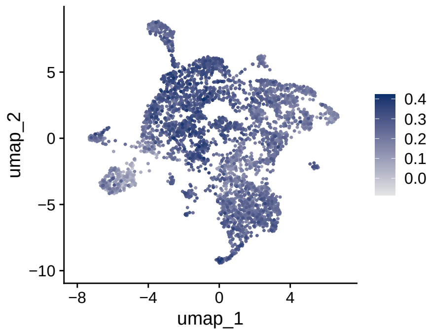
TJ_module
