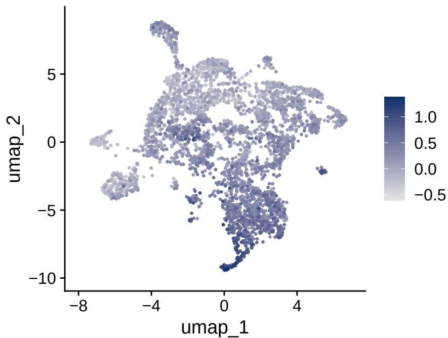
MHC_module
