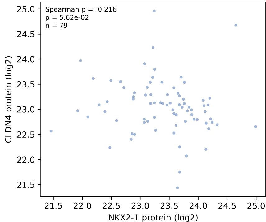
CPTAC-LUAD protein NKX2-1 vs CLDN4
