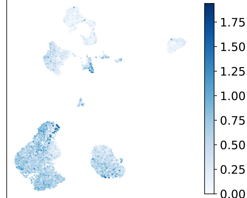
IFN ISG
