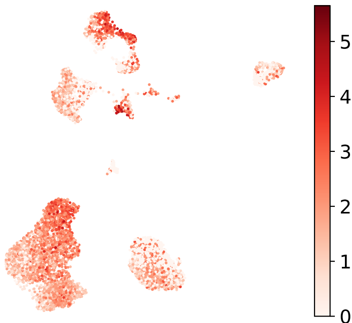
CLDN4
