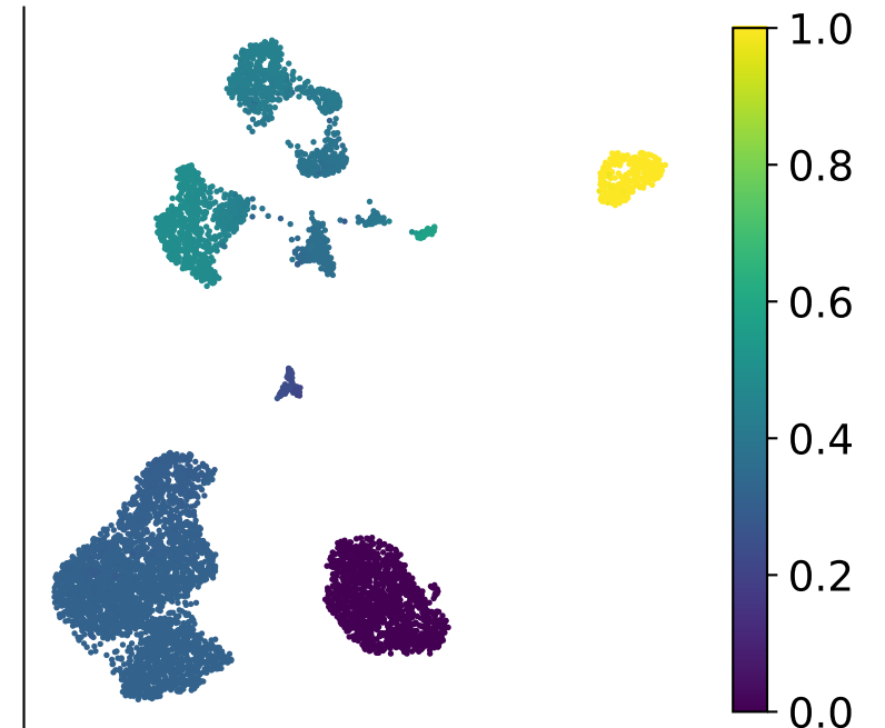
Palantir pseudotime
