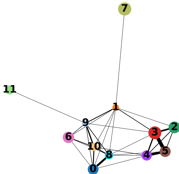
PAGA (Leiden)
