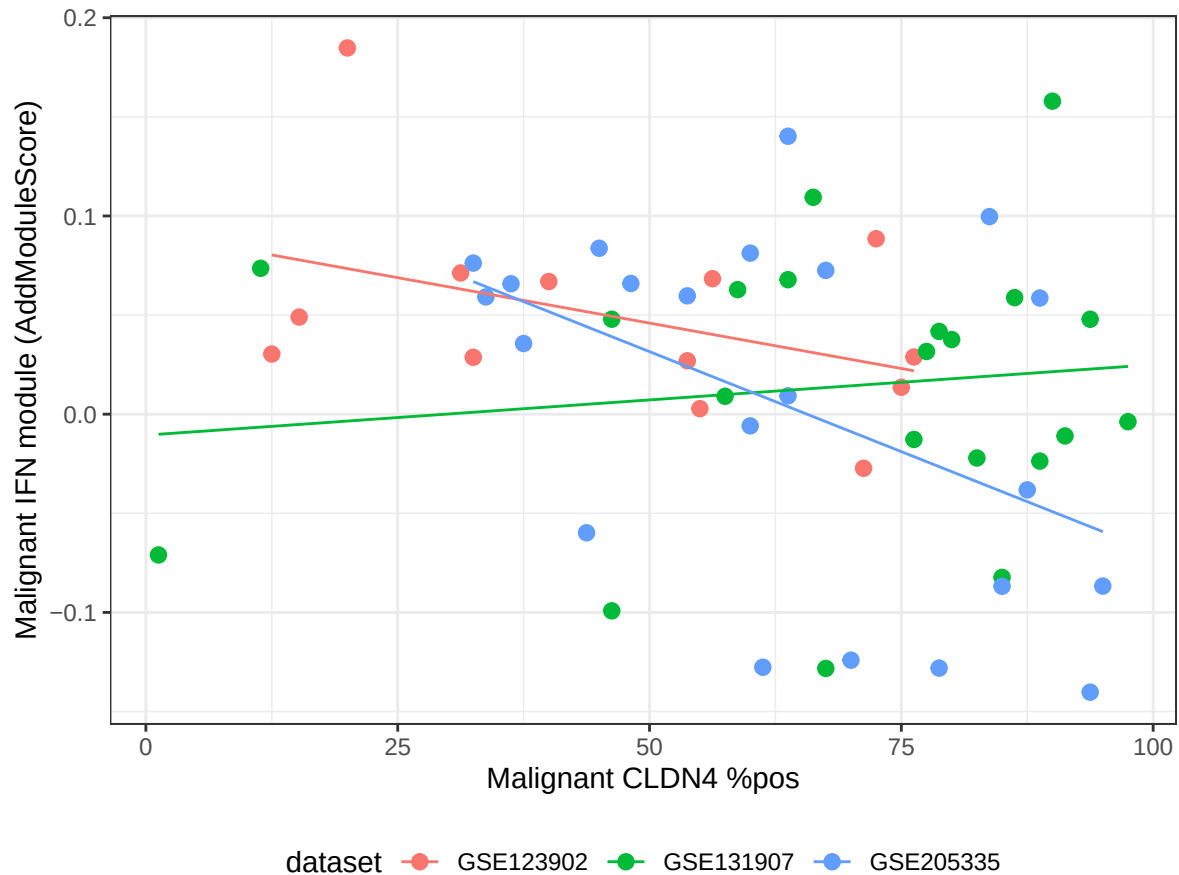
Patient unit: CLDN4 vs malignant IFN
