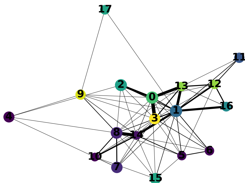
PAGA (Leiden) mean CLDN4
